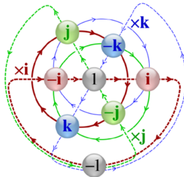
Рисунок 1 – Кватернион
