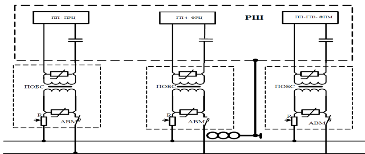
Рис. 1 – Схема включения элементов защиты рельсовых цепей тональной частоты при любом виде тяги
